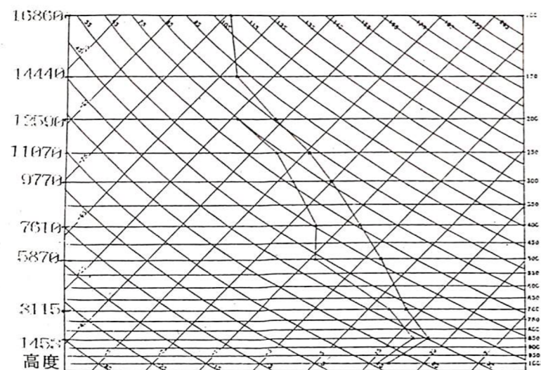
圖六 57494 測站 8月28日 00 Z 之斜溫圖
