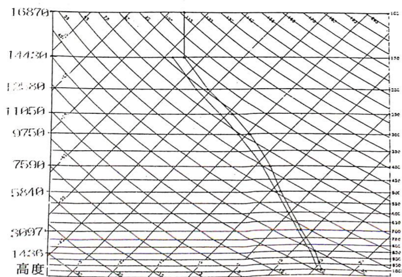
圖七 57494 測站 8月28日 12 Z 之斜溫圖
