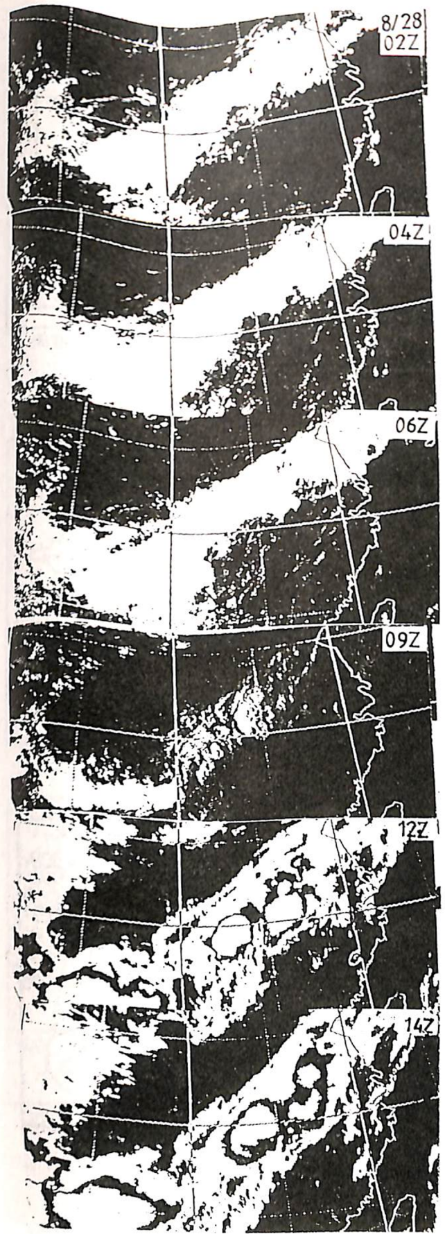
圖二 8月26~28日主要對流系統之移行及伴隨天氣現象
