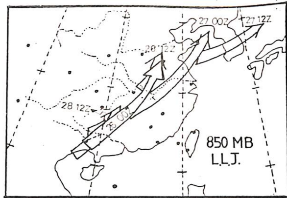
圖四 8月26日至28日850 mb 低層噴流示意圖
