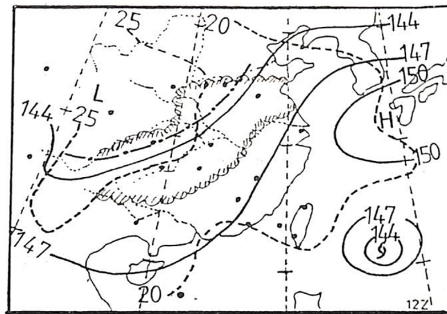
圖五 8月28日00Z及12Z之850 mb 天氣圖、雲圖示意圖，虛綫為等溫綫
