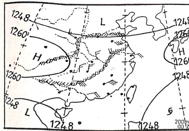
圖八 8月28日00Z及12Z之300 mb、200 mb 天氣圖及風場
