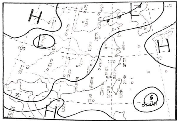
圖三 8月28日00Z地面天氣圖
