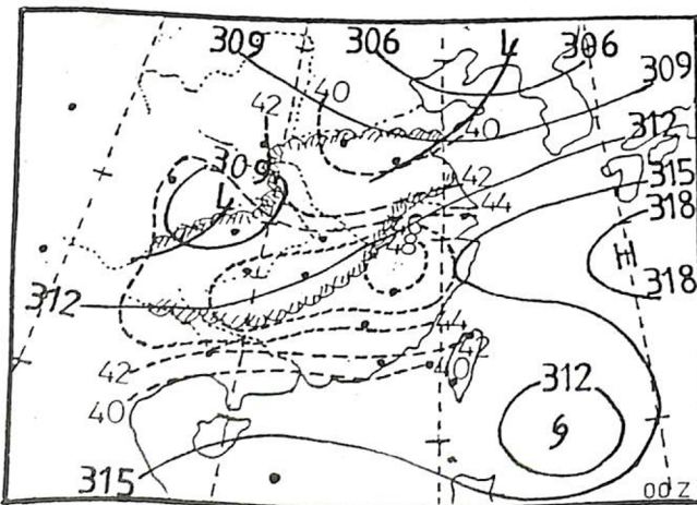
圖六 8月28日00Z及12Z之700 mb 天氣圖，實綫為等高綫，虛綫為K I
