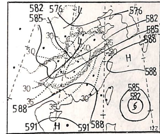
圖七 8月28日00Z及12Z之500 mb 天氣圖，實綫為等高綫，虛綫為K I
