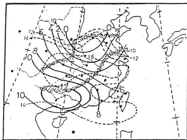
圖九 8月28日 00 Z, 實綫為 \theta_{e, 850mb} - \theta_{e, 500mb} 點綫為 850 mb 比濕
