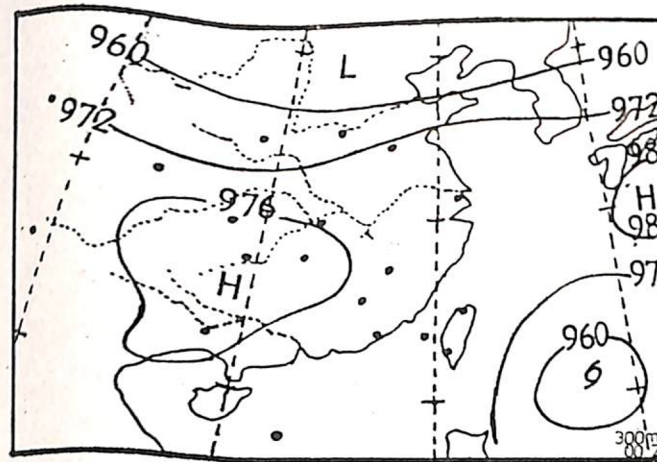
圖七 8月28日00Z及12Z之500 mb 天氣圖，實綫為等高綫，虛綫為K I
