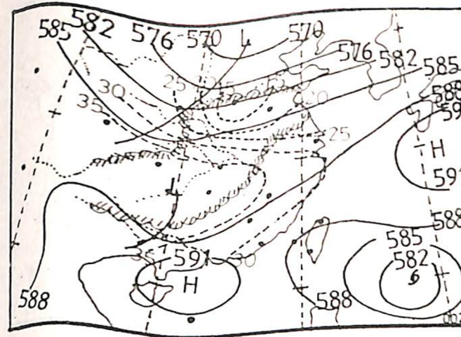
圖七 8月28日00Z及12Z之500 mb 天氣圖，實綫為等高綫，虛綫為K I
