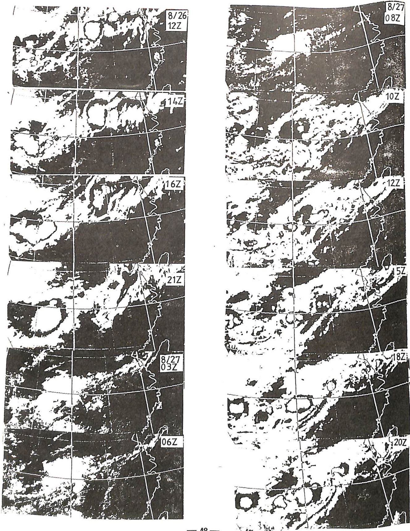
圖一 76年8月26日至28日GMS-3衛星雲圖
