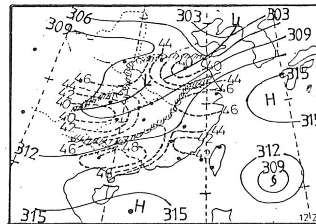
圖六 8月28日00Z及12Z之700 mb 天氣圖，實綫為等高綫，虛綫為K I
