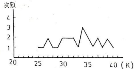
圖(八)75、76年綠島探空因子，K指數發生次數關係圖。
