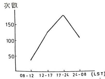
圖七 台東地區61~76年，歷年雷雨發生之時間統計曲線圖
