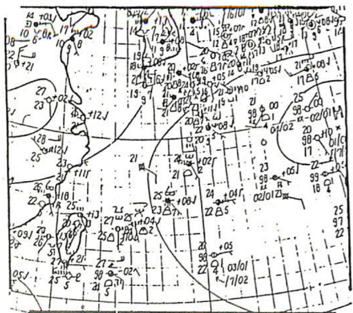
圖(五)民國70年5月8日12Z地面圖雷雨發生時之綜觀天氣型態太平洋高壓型。
