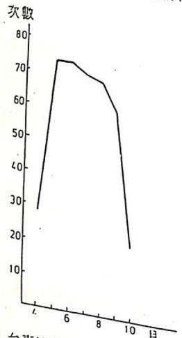
圖二 台東地區61~76年，4月至10月雷雨發生次數統計曲線圖。
