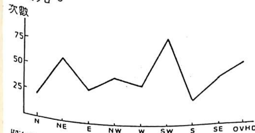
圖九 台東地區61~76年，歷年雷雨發生之方向統計曲線圖。
