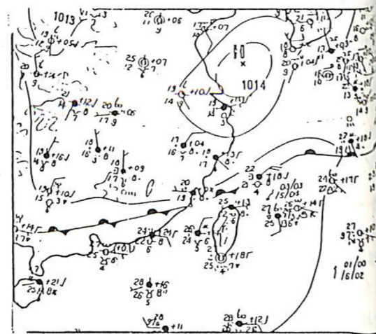
圖(七)民國67年6月1日00Z地面圖鋒前暖區型，颱風或熱帶低壓環流型，出現次數以五月份、八月份為最多，圖六為颱風環流型之資料，時間為民國63年6月17日12Z共雷雨發生時間從2345L至隔天18日的0310L，共計25分鐘，其綜觀天氣圖六。
