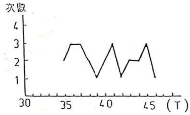
圖(七)75、76年綠島探空因子，T指數發生次數關係圖。
