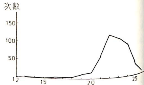
圖四 台東地區61~76年歷年雷雨發生當日最高溫度統計曲線圖。
