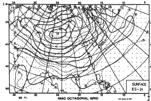
圖 2 c 極強寒潮前 24 小時地面合成圖。
