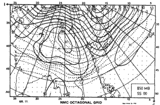
圖 6d 緩強寒潮過境時 850mb 合成圖。
