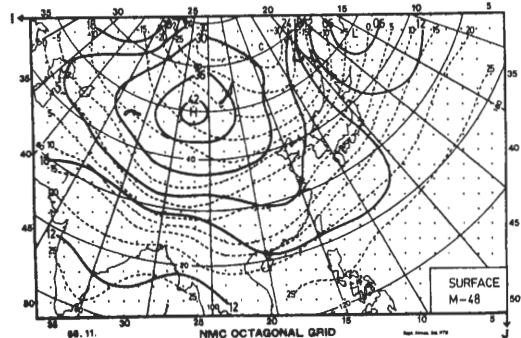
圖 1 a 冷鋒通過台灣北部地區前 48 小時，中寒潮地面合成圖，簡稱 M-48，負號表過境前，實線為等壓線 (mb)，虛線為等溫線 (°C)。以下各圖說明均同，不再重複。
