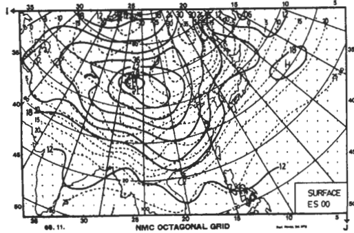
圖 3c 極強寒潮過境時地面合成圖。
