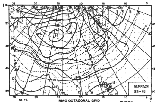
圖 1 d 緩強寒潮前 48 小時地面合成圖。
