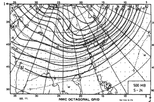
圖11b 強寒潮前24小時500mb合成圖。
