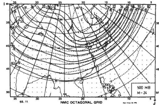
圖11a 中寒潮前24小時500mb合成圖。
