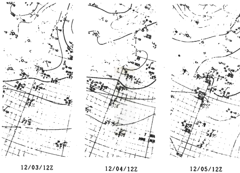
圖9 1986年12月3日至5日之地面天氣圖。圖中粗線為1020 mb等壓線。
