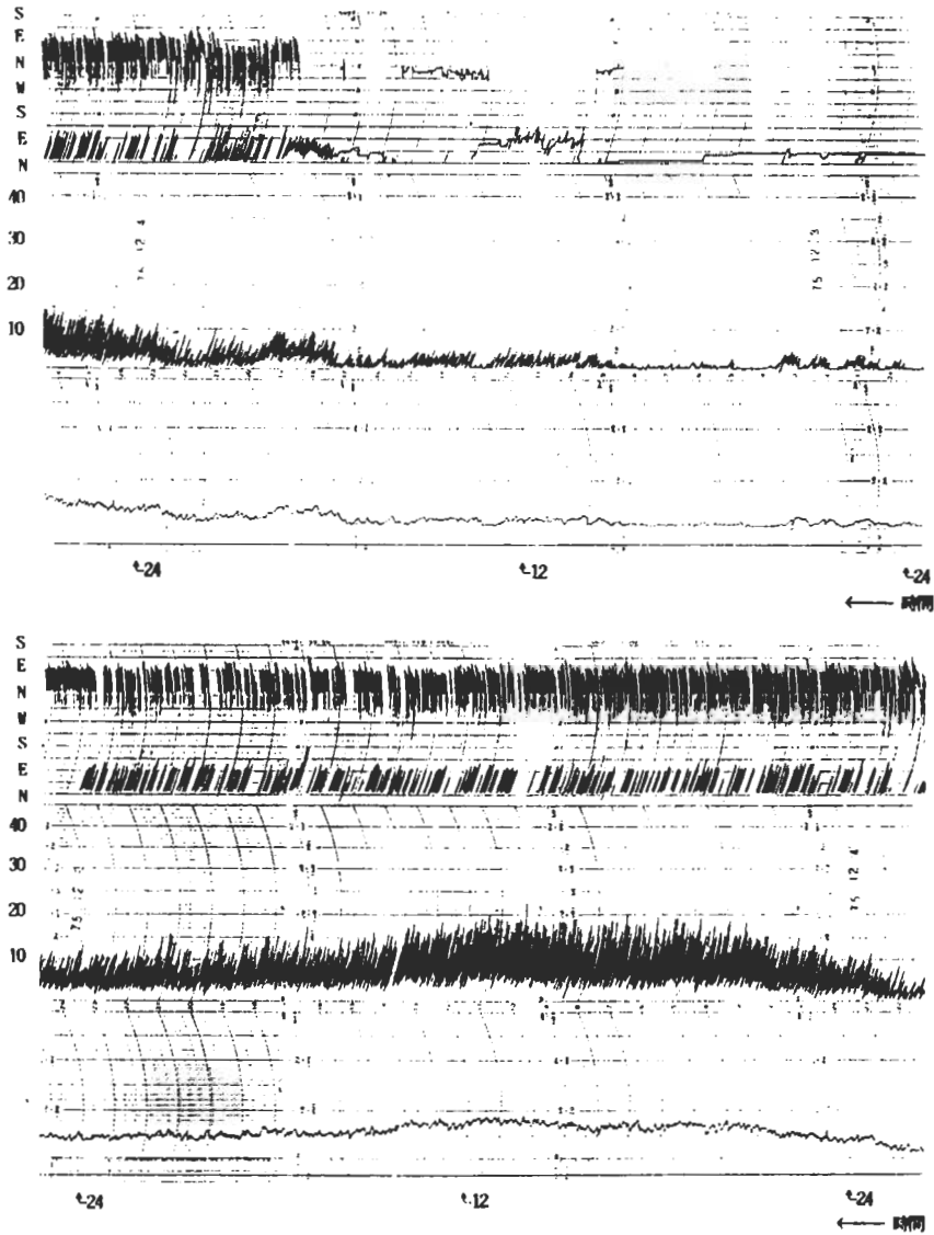
圖1 1986年12月3日至1日恆春測站之地面風速風向。
