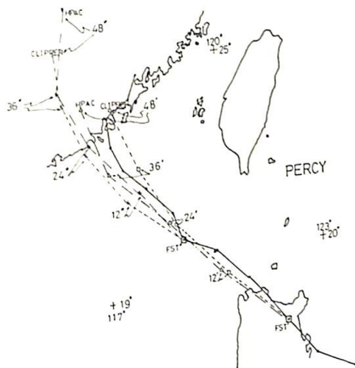
圖三：波西颱風路徑及在 FST' 與 FST'' 兩點時之 HPAC 與 CLIPPER 的路徑預報圖
