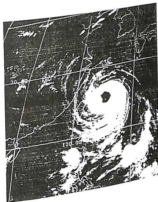
圖六：民國 79 年 8 月 29 日 GMS-04 2033 Z 紅外線加強雲圖，主要雲系為亞伯 (ABE) 颱風之雲系
