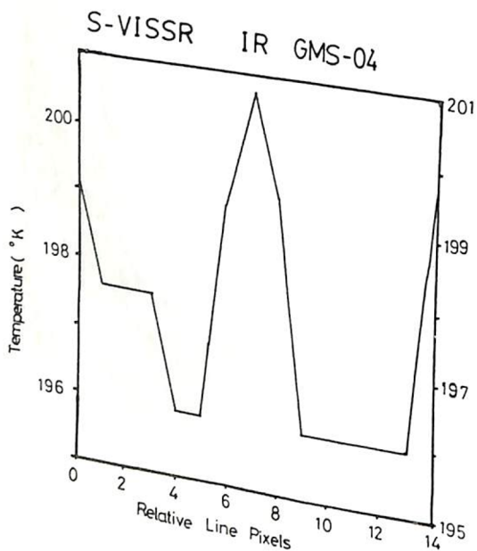
圖八：應用 GMS-04 S-VISSR IR 數據分析雲頂溫度的示意圖，雲圖時間為民國79年9月5日 2133 Z
