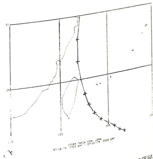
圖四：METPAK 中颱風路徑類型之製作，圖為民國63年7月16日至7月21日颱風珍恩 (JEAN) 的路徑示意圖。
