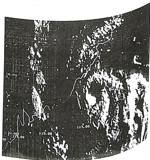
圖十：民國79年7月28日 2317 Z NOAA-10 AVHRR 可見光雲圖，主要雲系為波西颱風之雲系，此圖斜視誤差明顯。
