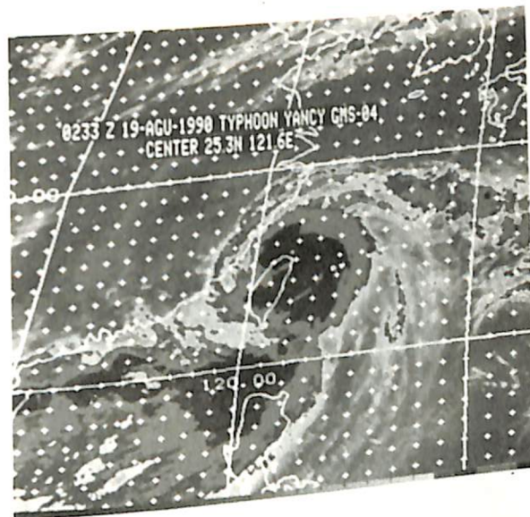
圖五：民國 79 年 8 月 19 日 GMS-04 0233 Z 紅外線加強雲圖，颱風楊希中心清晰可見
