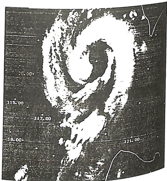
圖九：民國79年7月28日 0526 Z NOAA-11 AVHRR 可見光雲圖，主要雲系為波西颱風之雲系
