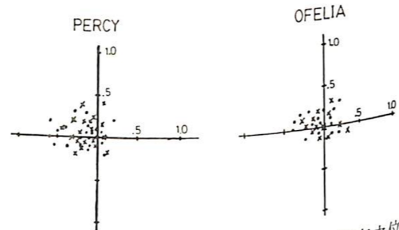
圖五：校驗波西與歐菲莉颱風位置與美軍發布之位置及美軍利用衛星定位之位置比較，0.5代表0.5緯度，圖中×代表美軍發布相對於本軍衛星定位之相關位置，●代表美軍衛星定位相對於本軍衛星定位之相關位置
