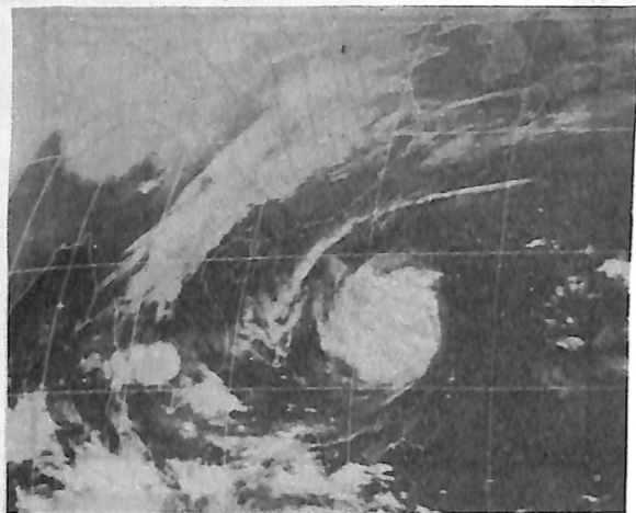
圖13.民國70年11月24日00z IR 衛星雲圖
