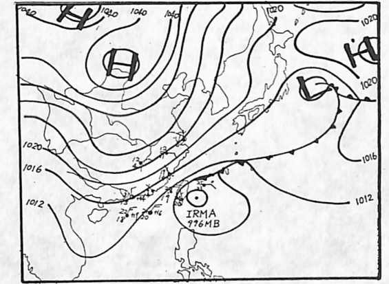
圖 10 民國 70 年 11 月 26 日 12z 地面天氣圖
