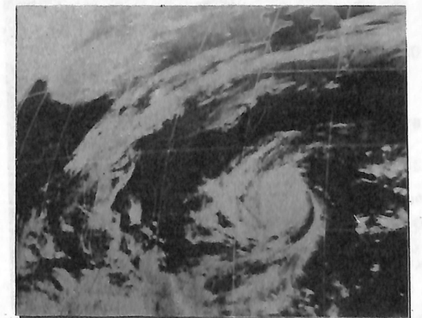
圖 12 民國 70 年 11 月 23 日 12z IR 衛星雲圖
