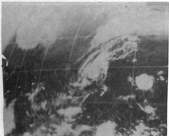
圖15.民國70年11月25日00z IR 衛星雲圖
