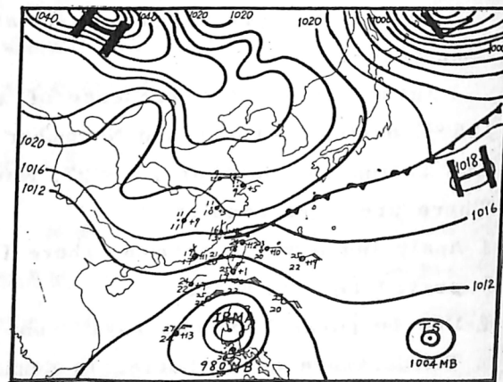
圖 6 民國 70 年 11 月 24 日 12z 地面天氣圖
