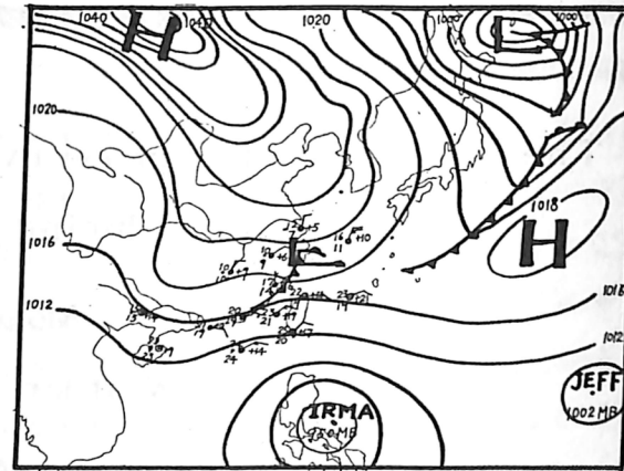
圖 5 民國 70 年 11 月 24 日 00z 地面天氣圖
