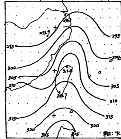
圖31.民國70年11月26日12z 850 MB 位溫分佈圖
