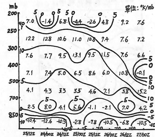
圖23.台北探空不穩定度時空剖面圖
