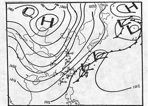
圖 11 民國 70 年 11 月 27 日 00z 地面天氣圖
