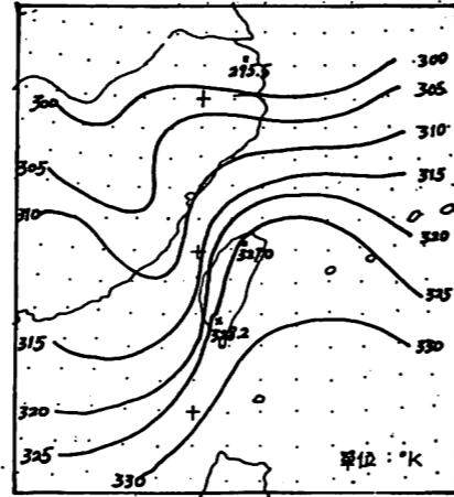
圖28.民國70年11月25日00z 850 MB 位溫分佈圖
