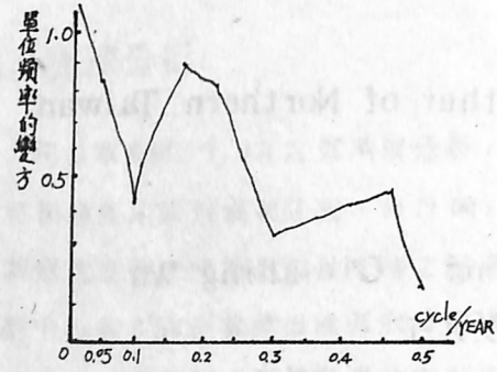
圖 2 10 月份颱風發生次數功率譜分佈圖
