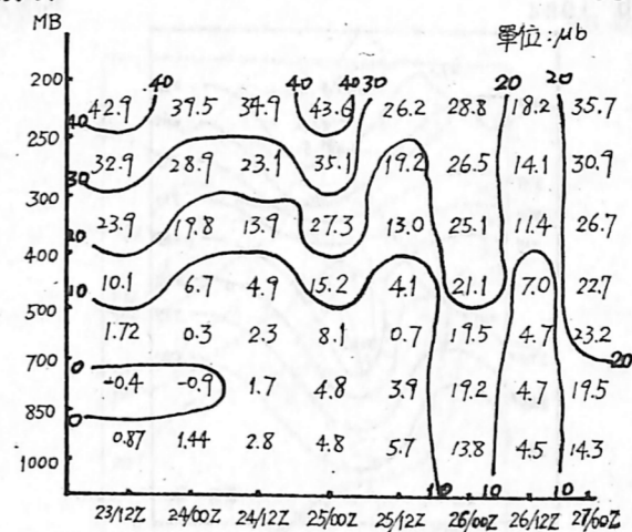
圖22.台灣區垂直速度時空剖面圖
