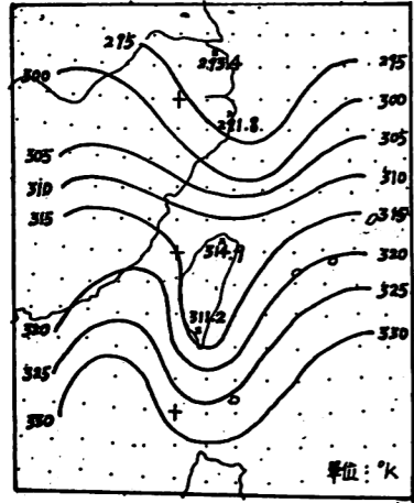
圖25.民國70年11月23日12z 850 MB 位溫分佈圖
