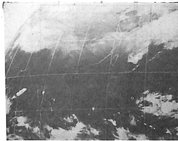
圖19.民國70年11月27日00z IR 衛星雲圖
