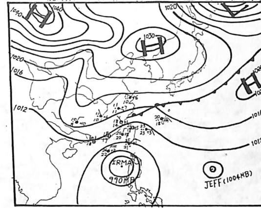
圖 7 民國 70 年 11 月 25 日 00z 地面天氣圖
