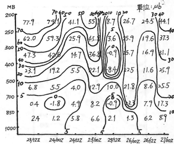
圖21.台灣海峽北部垂直速度時空剖面圖
