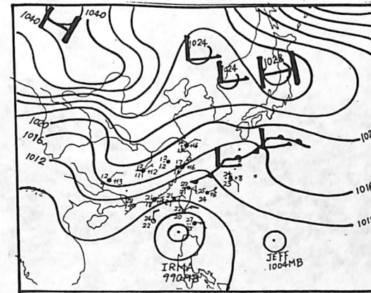
圖 8 民國 70 年 11 月 25 日 12z 地面天氣圖
