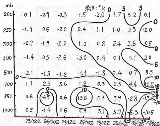
圖24.台北探空剖面位溫平均偏差圖
