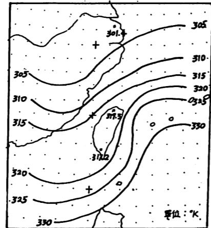
圖29.民國70年11月25日12z 850 MB 位溫分佈圖
