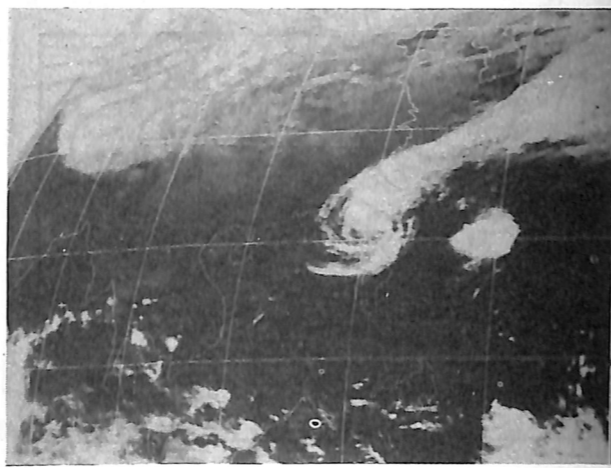
圖17.民國70年11月26日00z IR 衛星雲圖
