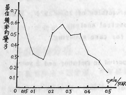
圖 3 11 月份颱風發生次數功率譜分佈圖
