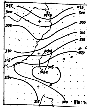
圖27.民國70年11月24日12z 850 MB 位溫分佈圖
