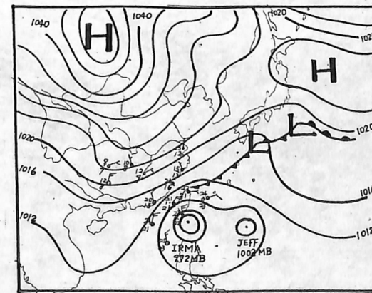
圖 9 民國 70 年 11 月 26 日 00z 地面天氣圖
