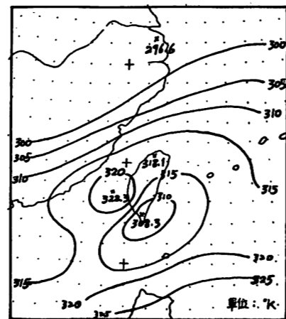
圖30.民國70年11月26日00z 850 MB 位溫分佈圖
