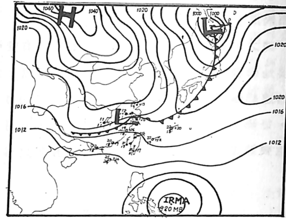
圖 4 民國 70 年 11 月 23 日 12z 地面天氣圖
