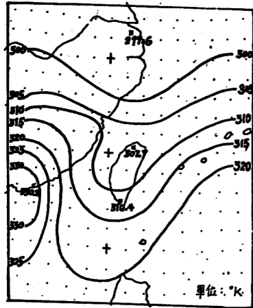
圖26.民國70年11月24日00z 850 MB 位溫分佈圖
