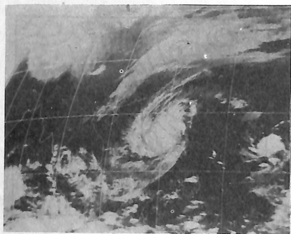
圖14.民國70年11月24日12z IR 衛星雲圖
