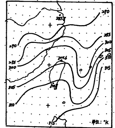
圖32.民國70年11月27日00z 850 MB 位溫分佈圖
