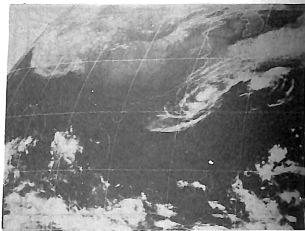
圖16.民國70年11月25日12z IR 衛星雲圖
