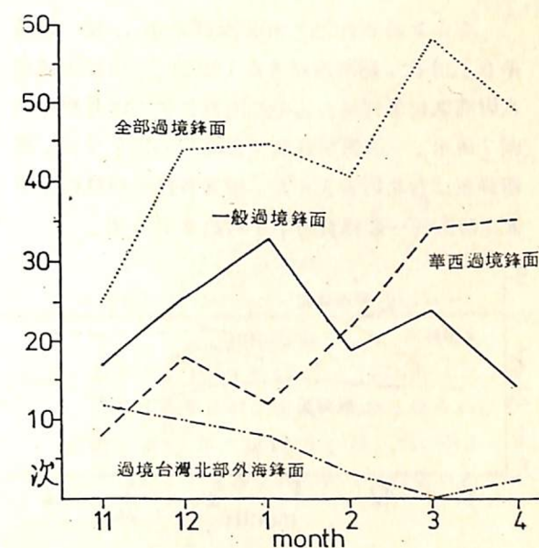
圖5：冬半年（1969年11月—1979年4月）十年間各類鋒面過境台北之鋒系次數逐月變化圖。
