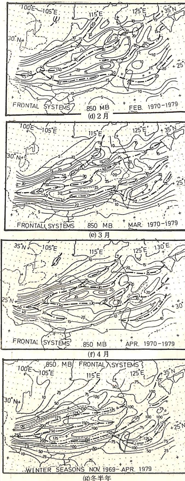
圖 13: 冬半年(1969年11月—1979年4月)逐月及冬半年在研究區域內850 mb風切線(鋒面)總頻率分布。(a)11月;(b)12月;(c)1月;(d)2月;(e)3月;(f)4月;(g)冬半年。
