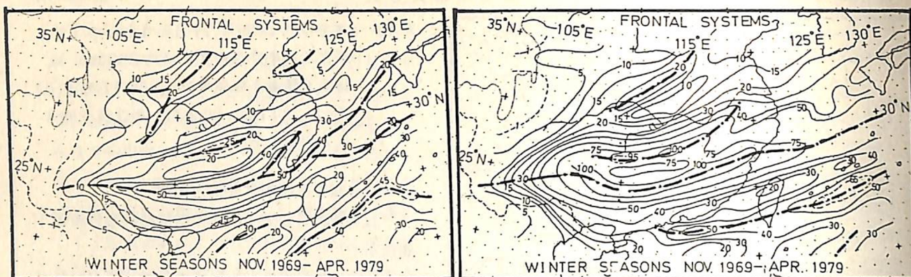
圖 15：冬半年（1969 年 11 月—1979 年 4 月）在研究區域內所出現過境台北之所有一般鋒面總頻率分布。
