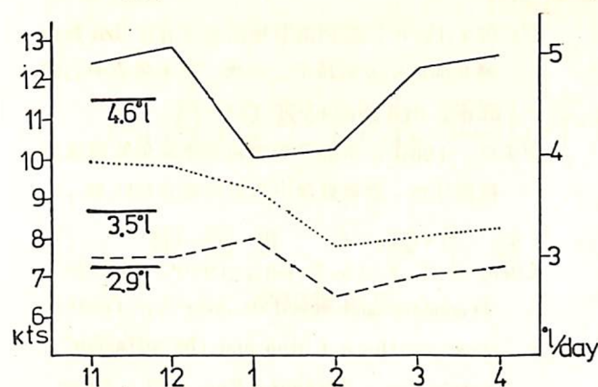
圖 17：冬半年（1969 年 11 月—1979 年 4 月）十年間逐月鋒面平均移速比較變化。（實線為一般過境鋒；虛線為華西過境鋒；點線為全部過境鋒。）
