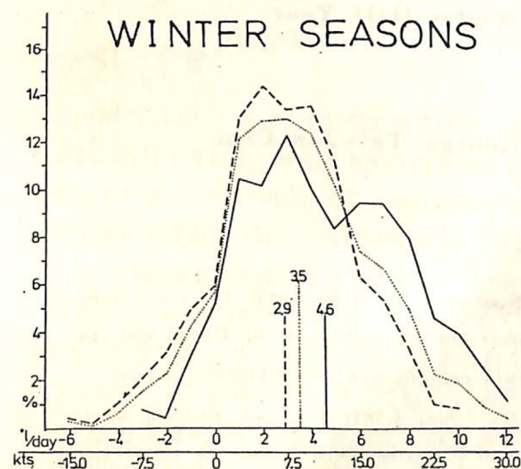
圖 18：（1969 年 11 月—1979 年 4 月）10 個冬半年間鋒面在研究區內移動至通過台北之各不同移速間距頻率分配。實線為一般過境鋒；虛線為華西過境鋒；點線為全部過境鋒。移速以緯度/天或哩/時，次數以%表示。
