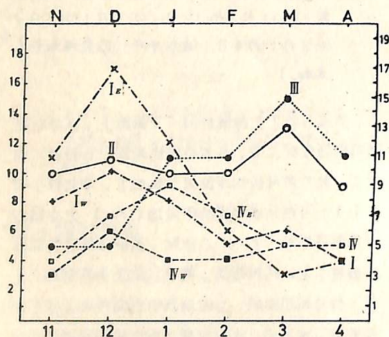
圖10：冬半年（1969年11月—1979年4月）研究範圍內逐月各鋒生帶鋒生次數變化圖。 。（×表華北鋒生（I：I s 漢中盆地；I w 渭河平原）；○表華中（長江）鋒生（II）；●表華南鋒生（III）；□表台灣附近鋒生（IV：IV s （□）台灣東方海面；IV w （■）台灣海峽。）
