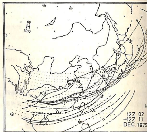
圖3：南類鋒且為華西鋒之實例。（實線為0000 GMT，斷線為1200 GMT）。
