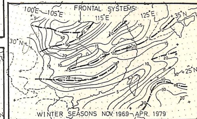
圖 14: 冬半年(1969年11月—1979年4月)在研究區域內所出現不過境台北之所有鋒面總頻率分布。
