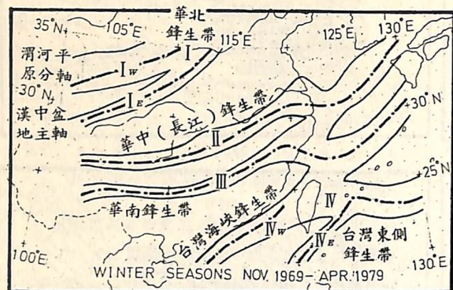
圖9：研究區域內逐月鋒生主軸範圍分布位置圖。 。斷點線表示冬半年鋒生主軸。
