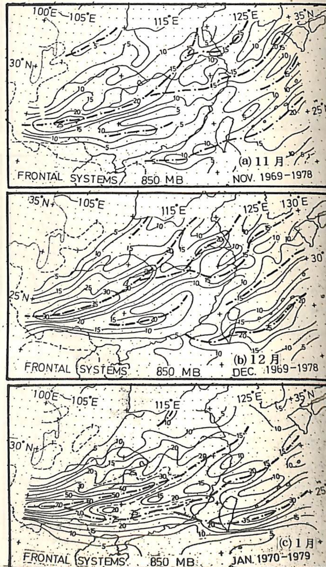
圖 12: 冬半年(1969年11月—1979年4月)研究範圍內逐月各區鋒面頻率最大次數變化圖。[×表華北鋒面(I); I E 漢中盆地; I W 渭河平原]; ○表華中鋒面(II); ●表華南鋒面(III); □表台灣附近鋒面(IV); IV E 台灣東方海面; IV W 台灣海峽。]
