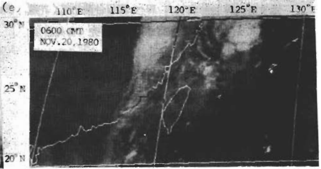
圖1 1980年11月18—20日GMS-1紅外線雲圖， (a) 18日0600 GMT，(b) 19日0600 GMT， (c) 19日1200 GMT，(d) 19日2100 GMT， (e) 20日0600 GMT。
