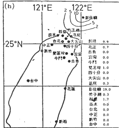
圖5 1980年11月19-20日每3小時降水量(公厘)分佈, 19日(a) 03-05 GMT, (b) 06-08 GMT, (c) 09-11 GMT, (d) 12-14 GMT, (e) 15-17 GMT, (f) 18-20 GMT, (g) 21-23 GMT, 20日(h) 00-02 GMT。
