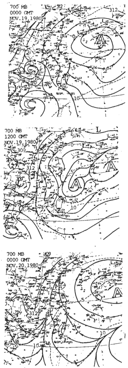
圖12 1980年11月19日00 GMT—20日00 GMT之 700 mb等高線 (dam) 氣流線與等溫線 (°C)
