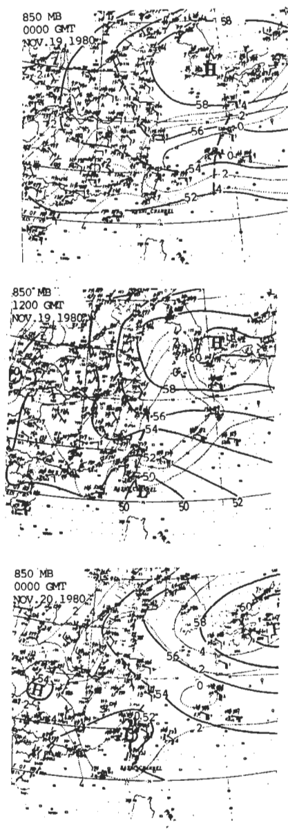
圖11 1980年11月19日00 GMT—20日00 GMT之 850 mb等高線 (dam) 與溫度—露點差 (°C) 分析。
