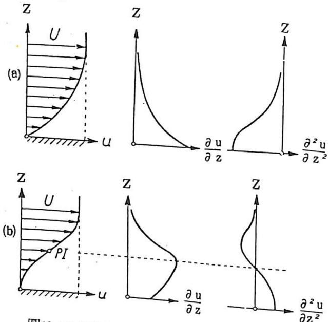
圖 10：(a) 氣壓隨高度遞減時之風速分佈。 (b) 氣壓隨高度增加時之風速分佈，PI 為反曲點。
