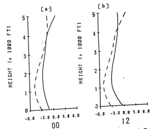
圖 4：台灣區平均風速分量 00 Z 與 12 Z 之垂直分佈 (a) 00 Z (b) 12 Z ( u 分量：實線， v 分量：虛線)
