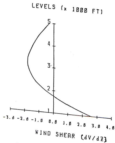
圖 11：台灣區平均風切之垂直變化
