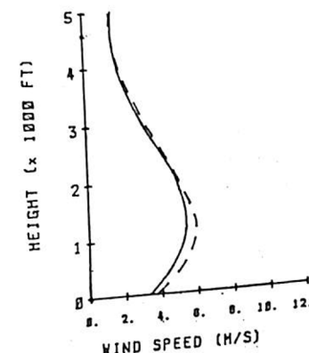
圖 5：台灣區 BL 內垂直風速 00 Z 與 12 Z 之比較 (00 Z：實線，12 Z：虛線)
