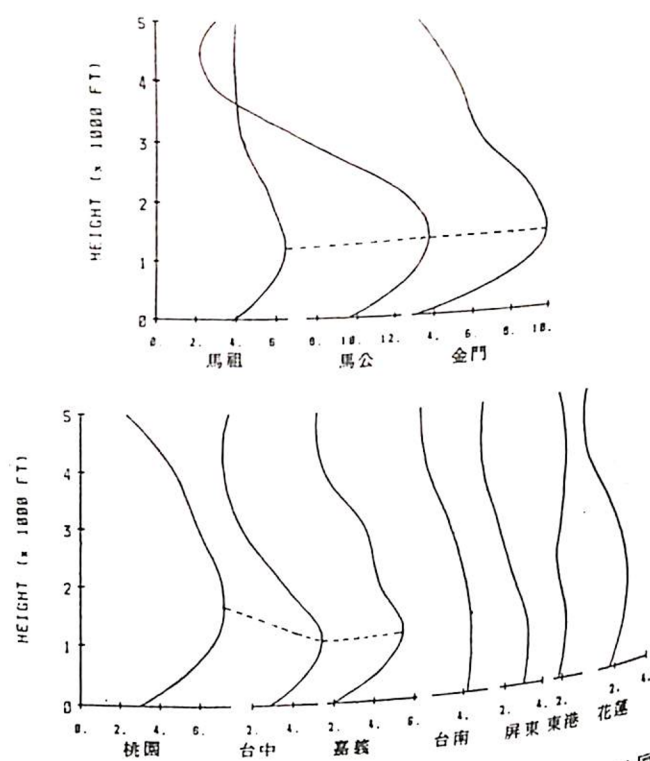
圖 8：台灣一月份平均風速垂直剖面圖及最大風層之高度變化
