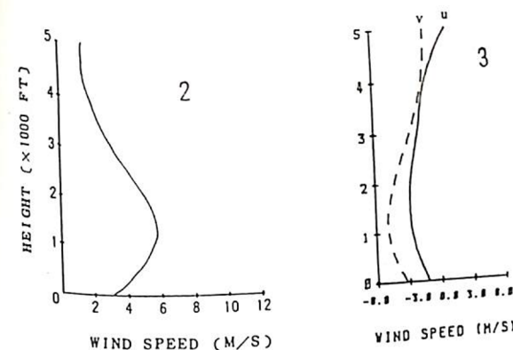
圖 2：台灣區邊界層內平均風速垂直剖面圖
