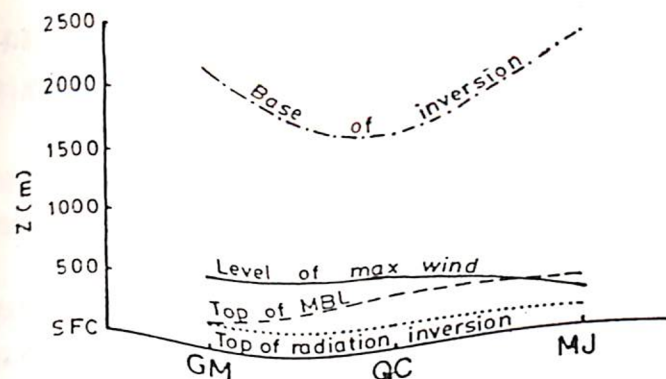
圖 15：台灣區冬季逆溫層，最大風層，混合邊界層 (MBL) 及輻射逆溫之高度分佈
