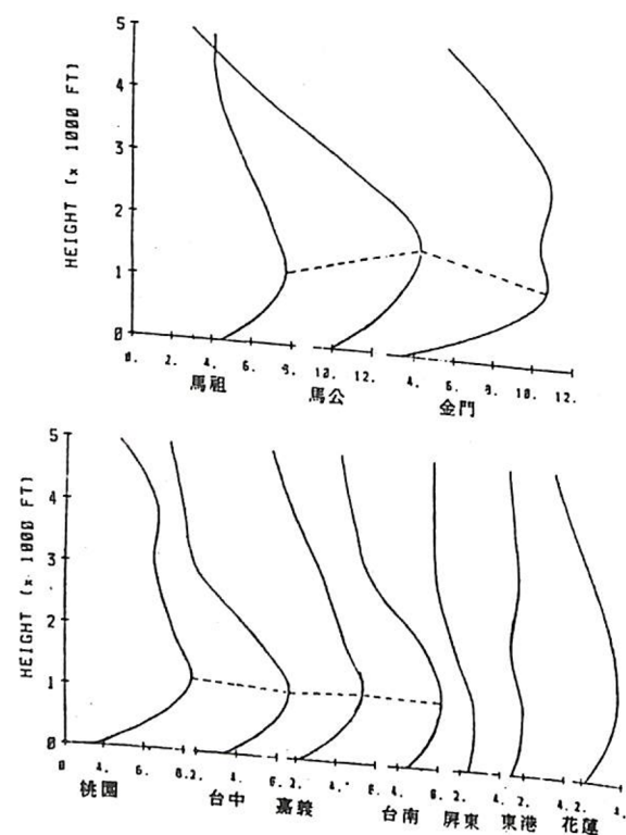
圖 7：台灣區十二月平均風速垂直剖面圖及最大風層之高度變化
