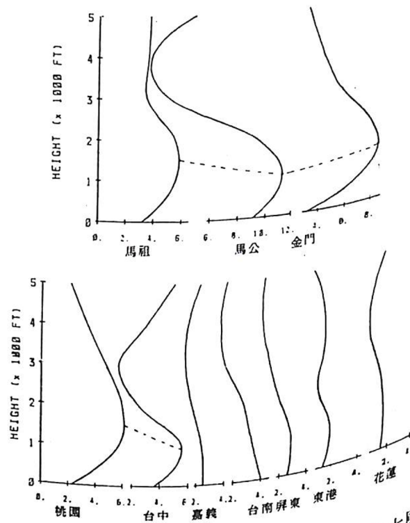
圖 9：台灣區二月份平均風速垂直剖面圖及最大風層高度變化
