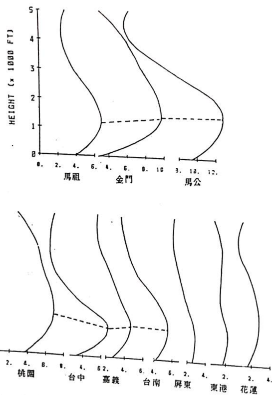
圖 6：冬季（12.1.2月）全省各站總平均垂直風剖面圖及最大風層之變化
