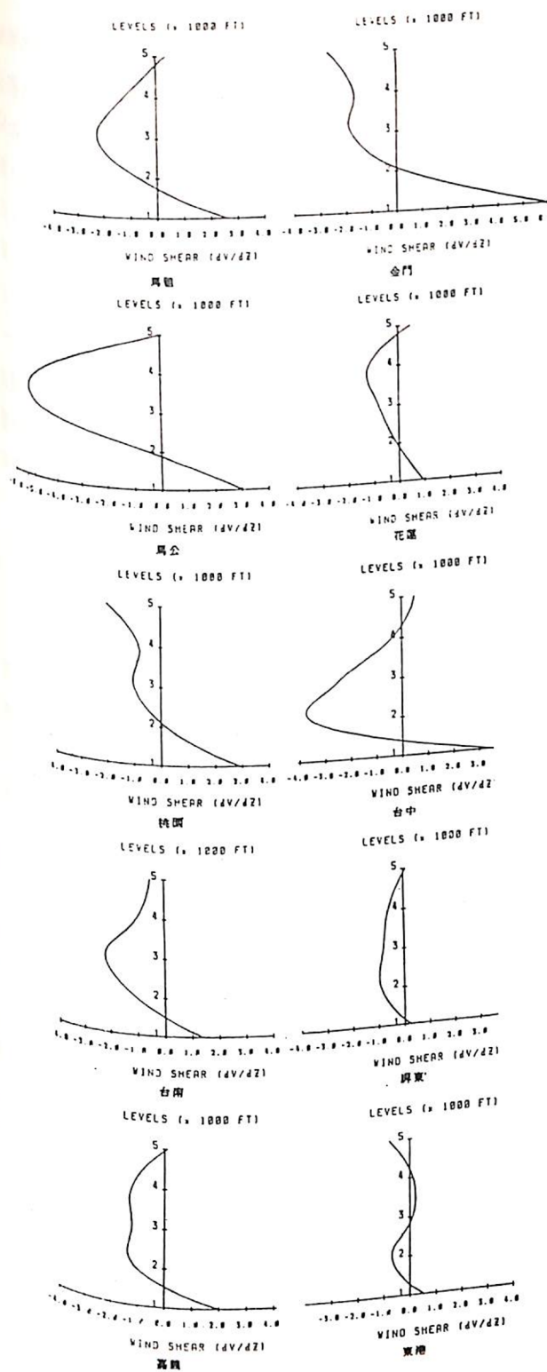
圖 12：台灣區各測站之風切垂直變化
