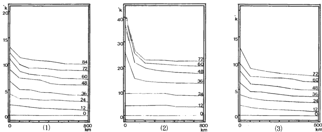
圖 7：第一部份實驗中，三個代表性的個案，其450MB位溫水平變差 ( \theta - 329.48^\circ\text{K} ) 在各時間隨著半徑的分佈
