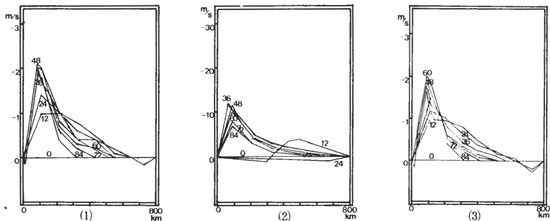
圖 6：第一部份實驗中，三個代表性的個案，其900MB徑向風的大小在各時間隨著半徑的分佈
