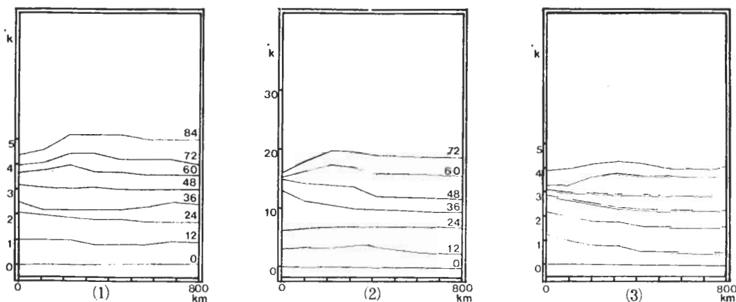
圖 8：第一部份實驗中，三個代表性的個案，其750MB位溫水平變差 ( \theta - 310.07^\circ\text{K} ) 在各時間隨著半徑的分佈
