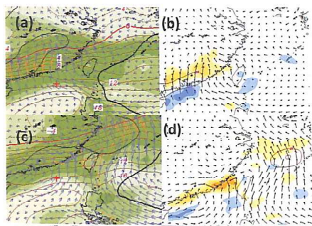
圖 5、同圖 4，但為 850hPa。
