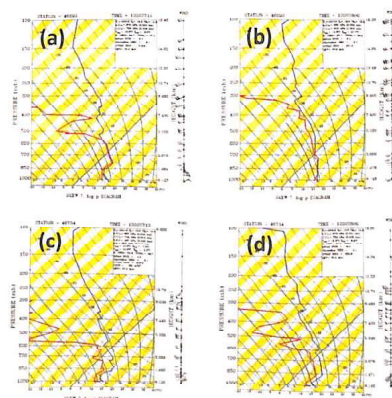
圖 11、板橋(46692)、馬公(46734)之探空資料，其中(a)、(c)為101年02月27日12Z，(b)、(d)為02月28日00Z。
