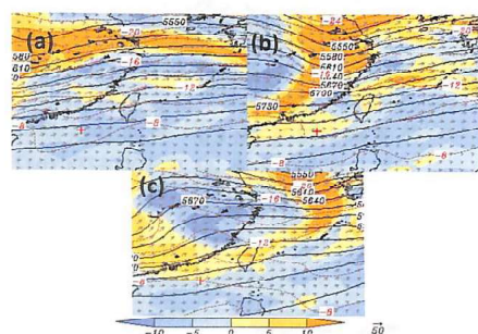
圖 6、500hPa 風場、溫度場、重力位高度、及渦度場，其中着色區為相對渦度，暖色系為正渦度，冷色系為負渦度、紅實線為溫度場、黑實線為重力位高度、箭頭為風標，時間分別為(a)101年2月27日12Z時(b)101年2月28日00Z時(c)101年2月28日12Z時。
