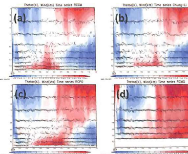
圖 13、模式模擬之2km以下相當位溫( \theta_e )及風場時間序列圖，模式網格解析度為1km，其中垂直方向風場(w)放大10倍，時間自101年02月28日00Z至12Z，各圖以各測站之經緯度為參考點，其中(a)參考點為桃園機場(RCGM)(b)參考點為中壢(c)參考點為新竹機場(RCPO)(d)參考點為清泉崗機場(RCMQ)。
