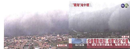
圖 1、中壢地區民眾於2012年02月28日下午拍攝到類似滾軸雲(roll cloud)之天氣現象(摘自網路)。
