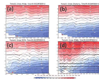
圖 12、模式模擬之2km以下位溫( \theta )及風場垂直剖面圖，模式網格解析度為1km，其中垂直方向風場(w)放大10倍，各圖以各測站之經緯度為參考點，切南北方向剖面，圖左側為南方，圖右側為北方，時間則選擇密度流大約抵達各測站時間，各圖中紅色三角形即代表各參考點位置，其中(a)為桃園機場(RCGM)、時間為1350時(b)為中壢、時間為1350時(c)為新竹機場(RCPO)、時間為1330時(d)為清泉崗機場(RCMQ)、時間為1430時。
