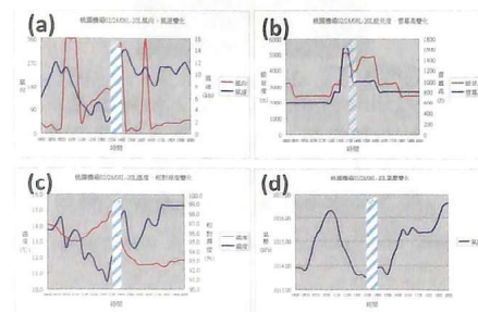
圖 7、桃園機場(RCGM)101年02月28日08時至20時各氣象要素變化，其中(a)紅線表示風向(°)、藍線表示風速(kts)(b)紅線表示能見度(m)、藍線表示雲幕高(ft)(c)紅線表示溫度(°C)、藍線表示相對溼度(%)(d)藍線表示氣壓(hPa)。圖中藍色區段時間為1340至1400時，研判約為密度流抵達該地區時間。
