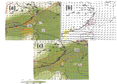
圖 4、925hPa 風場、溫度場、相對溼度、及輻合輻散場，其中左圖為相對溼度、紅實線為溫度場、黑實線為重力位高度、箭頭為風標，右圖為輻合輻散
