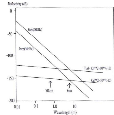
(圖二) 亂流與降水功率譜隨波長之分佈圖
