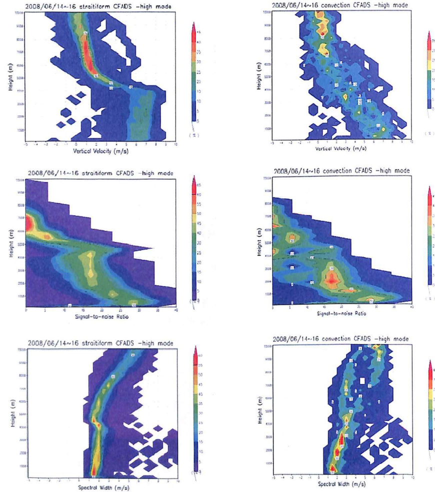
(圖六) 2008年6月14~16日，對流降水垂直速度、回波及頻譜寬隨高度統計圖。
