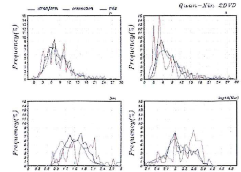
(圖七) 2008年6月14~16日中尺度對流系統，不同降水型態之 \mu 、 \Delta 、 D_m 、與 \log(N_w) 頻率分佈圖，黑線為層狀降水，紅線為對流降水，綠線為混合降水。
