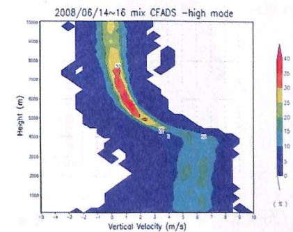
(圖四) 2008年6月14~16日，混合降水垂直速度、回波及頻譜寬隨高度統計圖。
