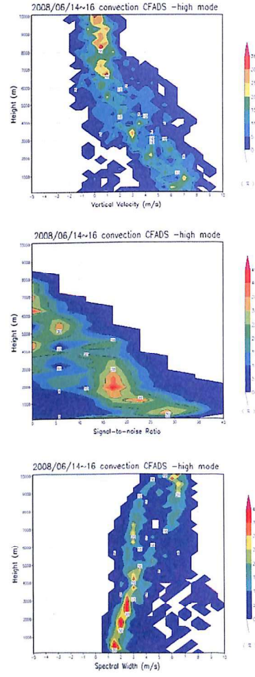
(圖六) 2008年6月14~16日，對流降水垂直速度、回波及頻譜寬隨高度統計圖。
