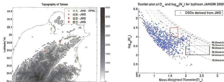
圖4 雨滴個數取對數(log 10 N w )與D m 散佈關係圖，橫軸表示D m 值，縱軸表示log 10 N w 值，紅（黑）色方框表示海洋（大陸）型對流降雨系統，虛線表示降雨率，間隔為10 mm hr -1 。
