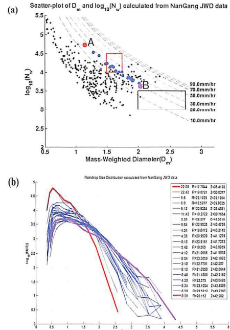
圖9 (a)南港雨滴儀觀測之 D_m-N_v 佈關係圖, 紅(A)、藍、粉紅(B)點為降雨率接近 20 \text{ mm hr}^{-1} ; (b)為(a)紅(A)、藍、粉紅點(B)對應雨滴粒徑分佈圖, 觀測資料時間、降雨率(R)與反射率(Z)如(b)右邊方框內所示。
