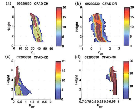
圖11 同圖10, 『B點』觀測資料時間為2008年9月28日0830 UTC。
