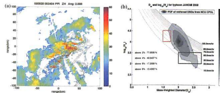
圖7 (a)2008年9月28日0034 UTC雷達 2.0^\circ 仰角PPI回波圖, 黑色方框為反演DSD範圍; (b)機率密度分布圖(PDF), 為(a)方框範圍反演結果, 灰階部分代表分布百分比。
