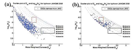
圖5 同圖4, (a)層狀降雨系統散佈圖, (b)對流降雨系統散佈圖。
