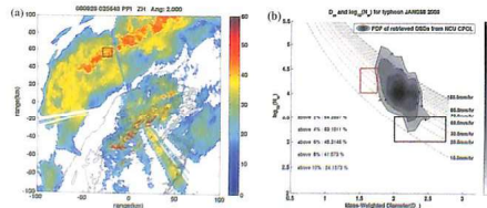
圖8 同圖7, 觀測資料時間為2008年9月28日0356 UTC。
