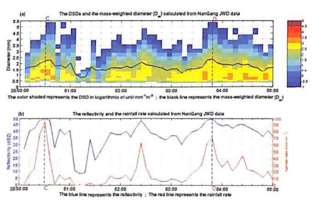
圖12 (a)為南港雨滴儀觀測雨滴粒徑分佈之時間序列圖, 縱軸表示雨滴等效體積直徑; 色階部份表示 N(D)(\text{mm}^{-1}\text{m}^{-3}) 值取對數( \log_{10} ), 黑色實線表示 D_m (mm)值。(b)為南港雨滴儀觀測資料計算降雨率及反射率之時間序列圖, 藍線為反射率(dBZ), 紅線為降雨率( \text{mm hr}^{-1} ), 左邊縱軸表示反射率, 右邊縱軸表示降雨率。(a)、(b)橫軸表示時間序列(UTC)。
