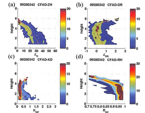
圖14 同圖10, 『D點』觀測資料時間為2008年9月28日0342 UTC。
