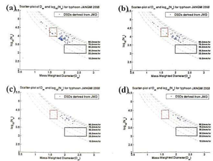
圖6 同圖4, (a)-(d)隨降雨率遞增 D_m-N_v 散佈關係圖, 遞增量間隔為 10 \text{ mm hr}^{-1} 。
