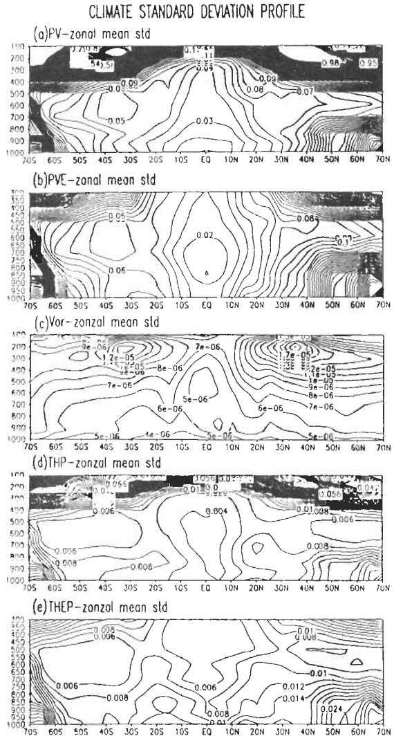
圖 2 為緯度圈平均的(a)位渦，(b)相當位渦，(c)絕對渦度，(d)靜力穩定度和(e)濕靜力穩定度的標準差的緯度-高度剖面圖。其中位渦和相當位渦的標準差的等值線間距為 0.01 PVU；絕對渦度的標準差的等值線間距為 10^{-6} \text{ s}^{-1} ；靜力穩定度和濕靜力穩定度的標準差的等值線間距為 0.002 \text{ }^{\circ}\text{K/hPa} 。
