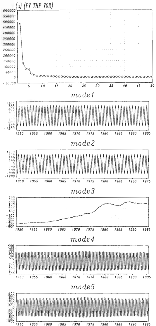
圖 6 由位渦、靜力穩定度和絕對渦度合成的 MSSA 分析所得的特徵值與前五個主分量。
