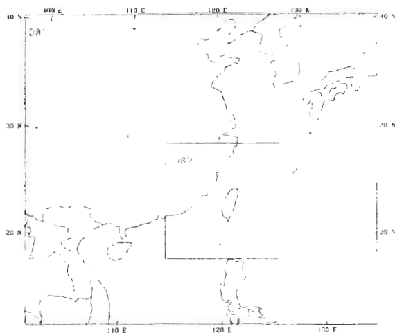
圖 3 MM5數值預報模式的網格設定，外層粗網格解析度為45km，網格點數為81x71；內層細網格的解析度為15km，網格點數為79x79。
