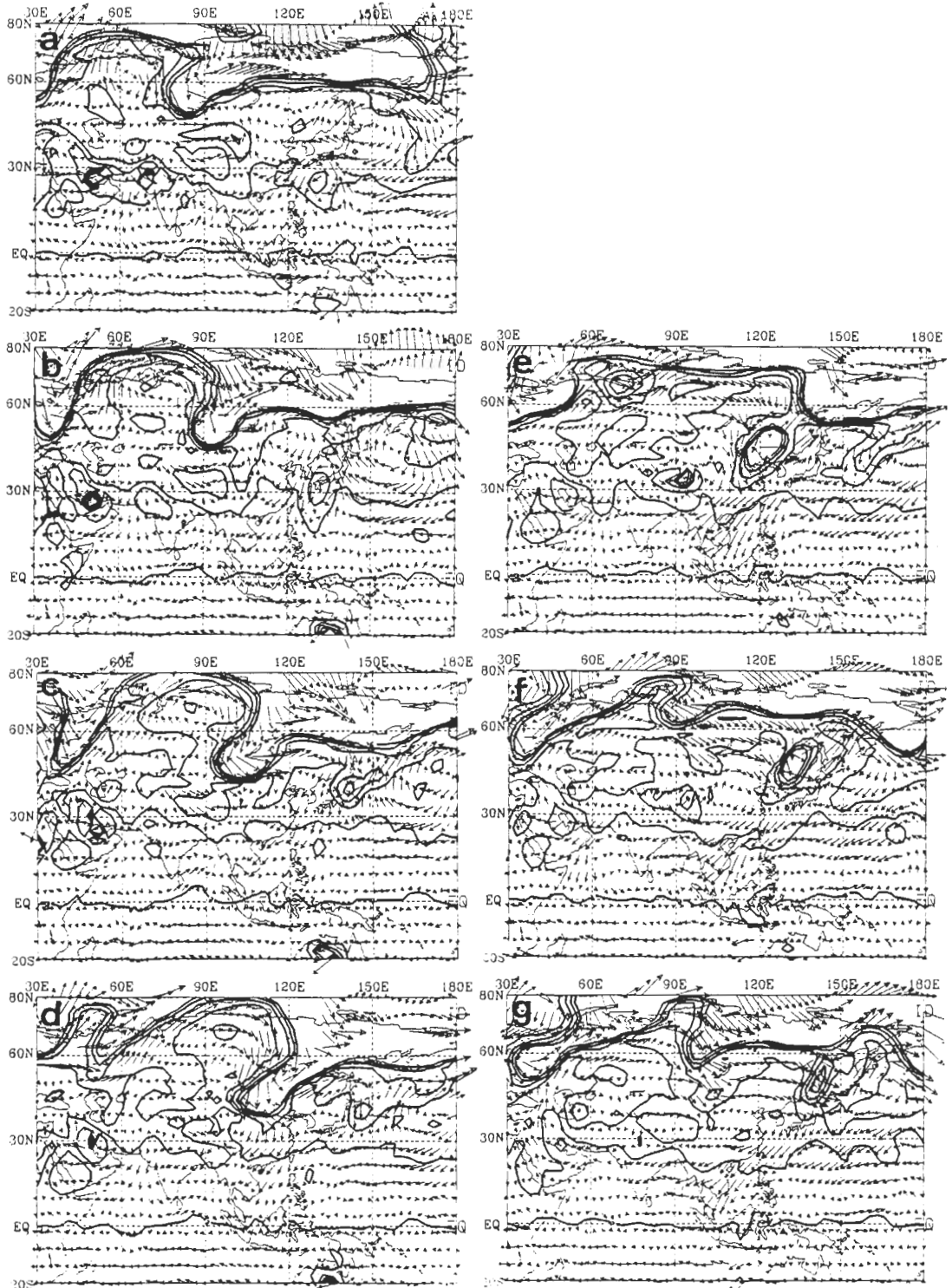
圖5 同圖4,但為300 k等位溫面上風場及IPV場,IPV數值自0至1.25,等值線間距為0.25,單位為 10^{-6}(k.m^2)/(s.Kg) ,(a)11月5日,(b)11月6日,(c)11月7日,(d)11月8日,(e)11月9日,(f)11月10日,(g)11月11日,1992年。
