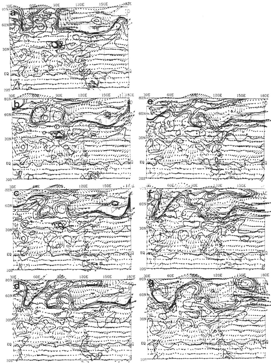
圖16 同圖6,但爲個案D, (a) 1月11日, (b) 1月12日, (c) 1月13日 (d) 1月14日, (e) 1月15日, (f) 1月16日及 (g) 1月17日, 1993年。
