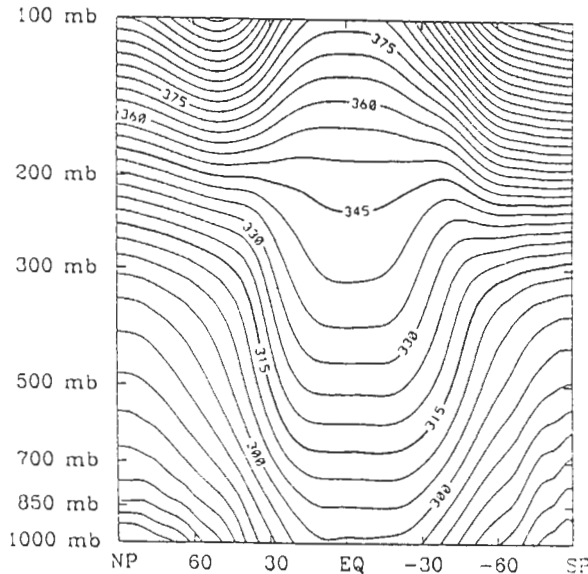
圖3 冬季(DJF)全球緯向平均等位溫之垂直分佈,摘自Thomas and Webster,1994
