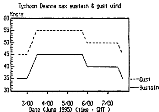
圖 1 - 2 : 荻安娜颱風之強度中心最大風速變化圖
