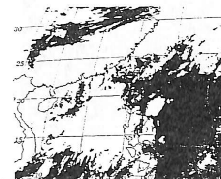
圖2-6：1995年6月8日0500時，經過強化處理後之衛星雲圖。
