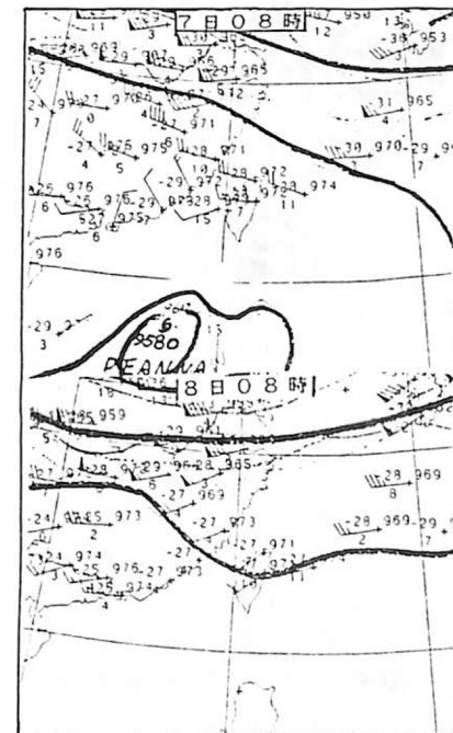
圖 4-5：1995年6月7日08時8日08時之300H PA天氣圖。
