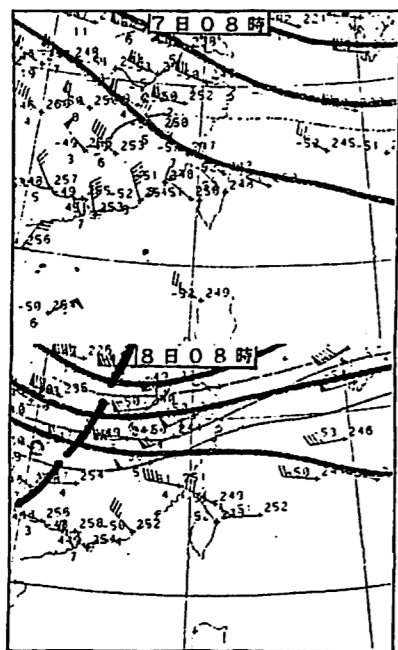
圖 4 - 6 : 1995年6月7日08時8日08時之200H PA天氣圖。
