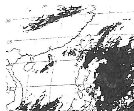
圖2-5：1995年6月8日0400時，經過強化處理後之衛星雲圖。
