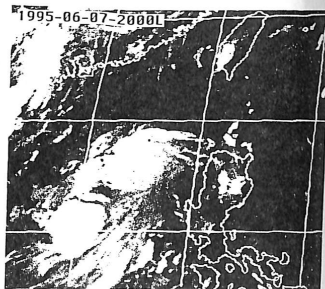
圖2-1：1995年6月荻安娜颱風移動之連續變化衛星雲圖
