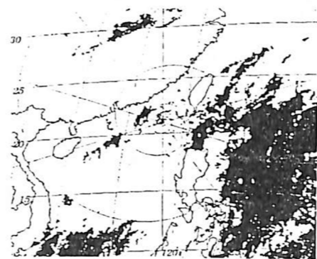
圖2-3：配合Dvorak之颱風中心定位。
