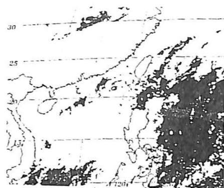
圖2-2：1995年6月8日0200時，經過強化處理後之衛星雲圖。
