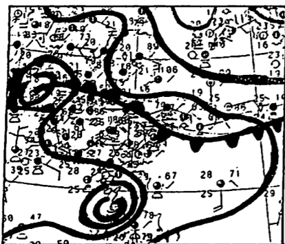
圖 5 - 1 : 1995年6月7日08時地面天氣圖。
