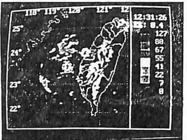
圖 3-3：1995年6月8日12時31分之雷達回波分析圖。
