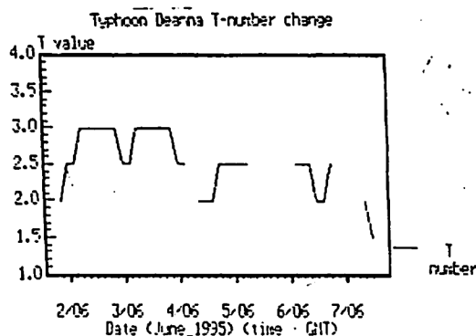
圖 1 - 1 : 荻安娜颱風之T-number值變化圖
