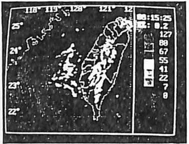
圖 3-2：1995年6月8日8時15分之雷達回波分析圖。
