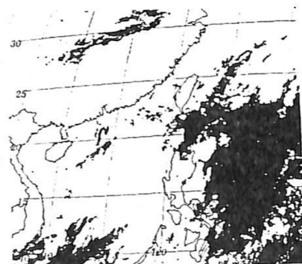
圖2-4：1995年6月8日0300時，經過強化處理後之衛星雲圖。
