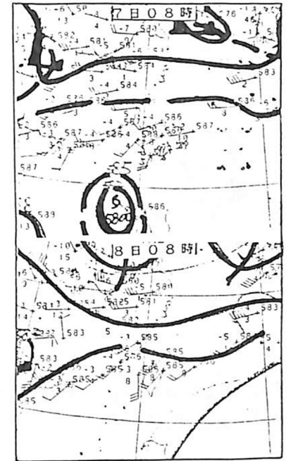
圖 4-4：1995年6月7日08時8日08時之500H PA天氣圖。
