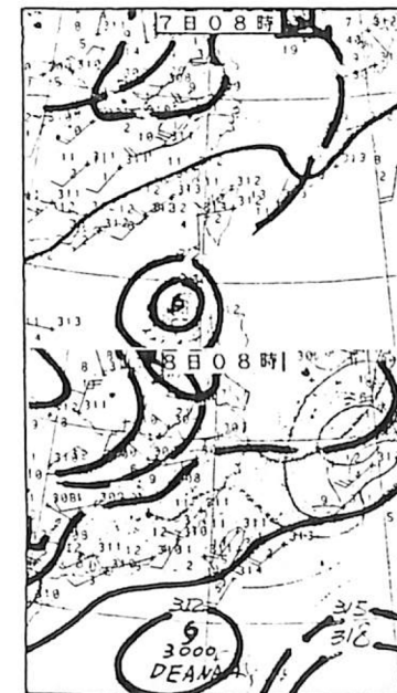
圖 4-3：1995年6月7日08時8日08時之700H PA天氣圖。
