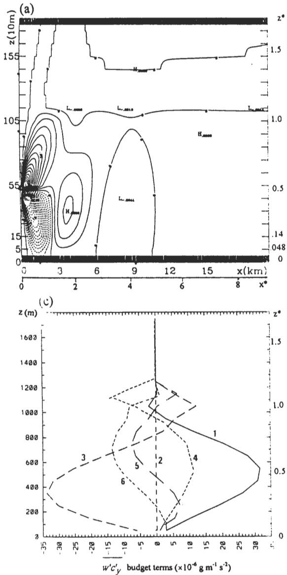
圖9 Day-34, 14時的(a) 無因次濃度通量 \overline{w'c'_y} 分布，等值線由-0.15至0.15，間格0.01，(b)在 x^*=0.5 的濃度通量收支：曲線1，平流項 -U(\overline{\partial w'c'_y / \partial x}) ；曲線2，水平梯度產生項 \overline{w'(\partial C_y / \partial x)} ；曲線3，垂直梯度產生項 -\overline{w'^2(\partial C_y / \partial z)} ；曲線4，互變異項 (g/\theta_0)(1-\alpha_2)\overline{c'\theta'_y} ；曲線5，擴散項 A\partial\{\sqrt{2E\lambda}(\overline{\partial w'c'_y / \partial z}) / \partial z\} ；曲線6，壓力項 -\alpha_1(\sqrt{2E/\lambda})\overline{w'c'_y} ，(c)同(b)但在 x^*=2.9 。坐標說明同圖8。
