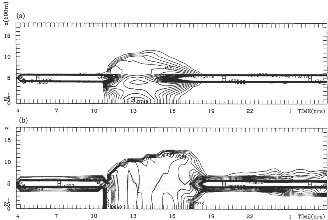
圖18 平均濃度 C_y(\text{g m}^{-2}) 的高度-時間變化：(a)在 x=2 公里，(b) 在 x=10.5 公里。等值線由0至0.45，間格0.015。等值線由0至0.21，間格0.007。
