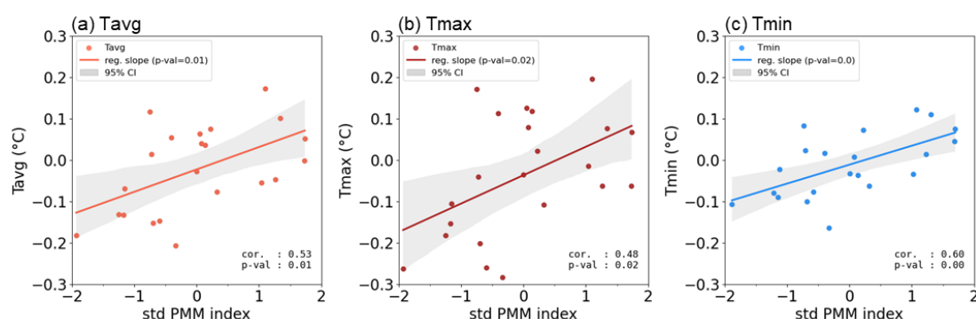
圖 5：臺灣在 1998-2022 年間夏季全島平均之日平均溫度、日最高溫度、日最低溫度與標準化 PMM 指數之散布關係。圓點在 (a) 為全台灣所有網格點，在五年滑動平均處理過後之日平均溫度（圖中標示為 Tavg），(b)、(c) 的資料處理與 (a) 相同，但分別日最高溫度（圖中標示為 Tmax）和日最低溫度（圖中標示為 Tmin），單位：°C。灰色陰影為 95% 信賴區間（Confidence Interval；CI）。資料年份為 1998-2022 年夏季。
