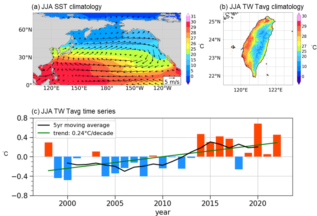
圖 1：(a) 1998 年至 2022 年夏季 (JJA) 太平洋區域海溫 (色階，單位：°C) 與 10 m 風場 (黑色箭頭) 之分布，可見副熱帶高壓下熱帶與副熱帶區域較高的海溫；(b) 同期臺灣平均溫度分布 (單位：°C)，顯示高溫主要集中在北部、西部及低海拔平原；(c) 1998 年至 2022 年臺灣夏季平均氣溫距平 (紅色長柱表示正距平、藍色長柱表示負距平)，並繪有 5 年移動平均 (黑線) 及長期趨勢線 (綠線)，其線性趨勢約為每十年上升 0.24°C，顯示臺灣夏季溫度持續有緩增的傾向。
