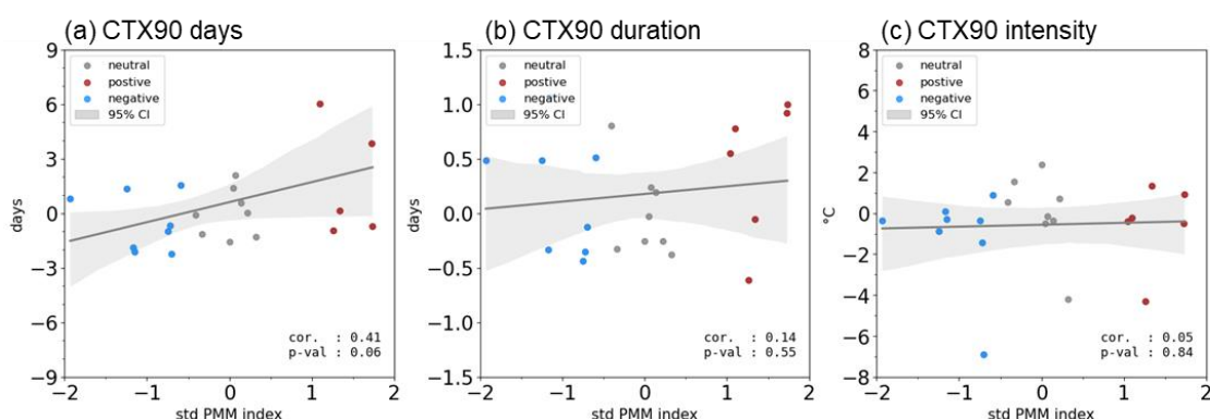
圖 10：臺灣夏季熱浪每年總天數、每次持續時間、每次平均強度與標準化 PMM 指數之間的散布關係。灰色圓點為 PMM 中立年、紅色圓點為 PMM 正向為年、藍色圓點代表 PMM 負相位年，圓點在 (a) 為熱浪每年總天數、(b) 為每次持數時間、(c) 為每次平均強度，單位： ^{\circ}\text{C} 。灰色陰影為 95%信賴區間（Confidence Interval；CI）。
