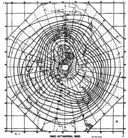
圖 13. 1967 年 12 月至 1977 年 2 月共十個冬季之平均 850mb 天氣圖。
