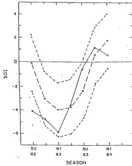
圖1 以單變數時間序列AR(3)模式所做Tahiti 減 Darwin氣壓差之季南方振盪指數 (SOI) 預報結果。SU82表示1982夏季，W183表示1983年冬季，實線表示觀測值，長斷線預測值，短斷線95%的可信賴區。Chu and Katz (1985)
