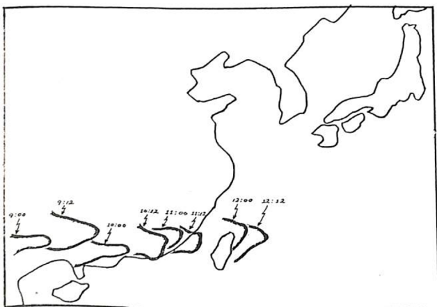
圖 6 1986 年 5 月 9 日至 12 日降水分布移動路徑，各箭頭所指為降水移動路徑之前緣。
