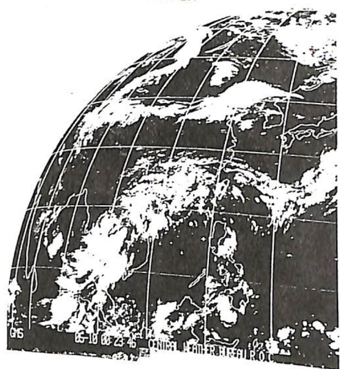
圖2-5 1986年5月10日00Z
