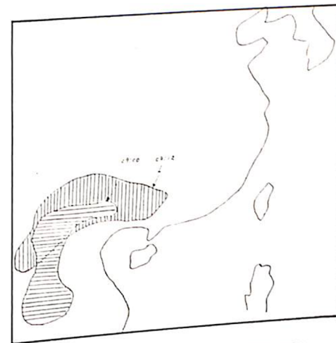
圖5-1 5月9日00Z及12Z
