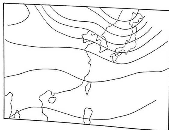
圖 8-4 5月12日 00 Z 500 mb 天氣圖
