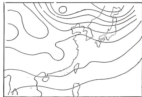
圖 7-4 5月12日 00 Z 700 mb 天氣圖
