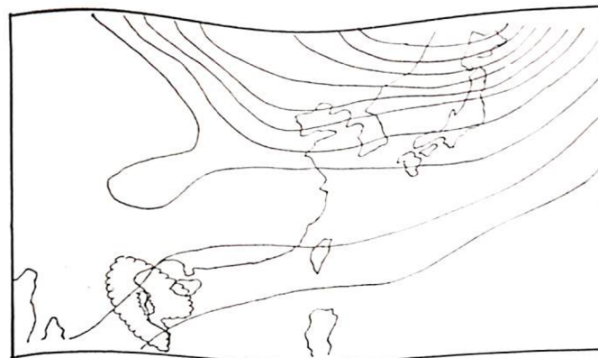
圖 7-2 5月10日 00 Z 700 mb 天氣圖
