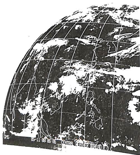
圖2-6 1986年5月11日00Z
