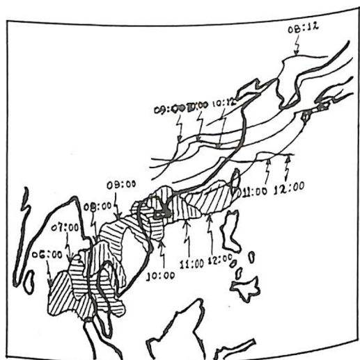
圖3 熱帶擾動雲系移動路徑及鋒面移動路徑連續圖。 斜線代表熱帶擾動雲系移動之前緣。
