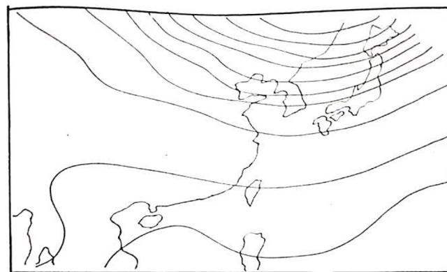
圖 8-2 5月10日 00 Z 500 mb 天氣圖
