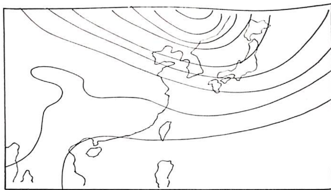
圖 7-1 5月9日 00 Z 700 mb 天氣圖
