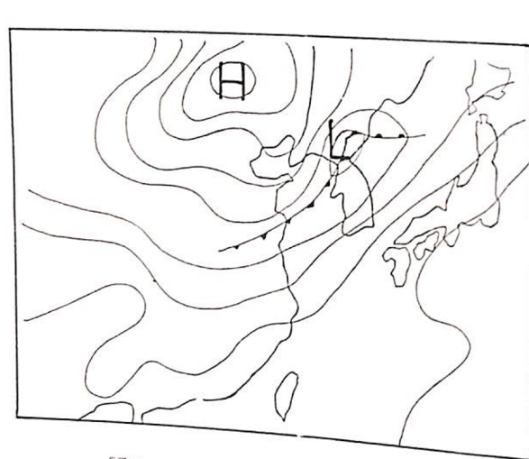
圖 1-1 1986年5月8日12Z天氣圖。
