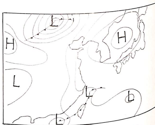
圖 1-4 1986年5月12日00Z天氣圖。
