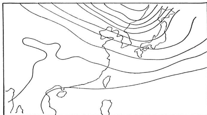
圖 8-1 5月9日 00 Z 500 mb 天氣圖
