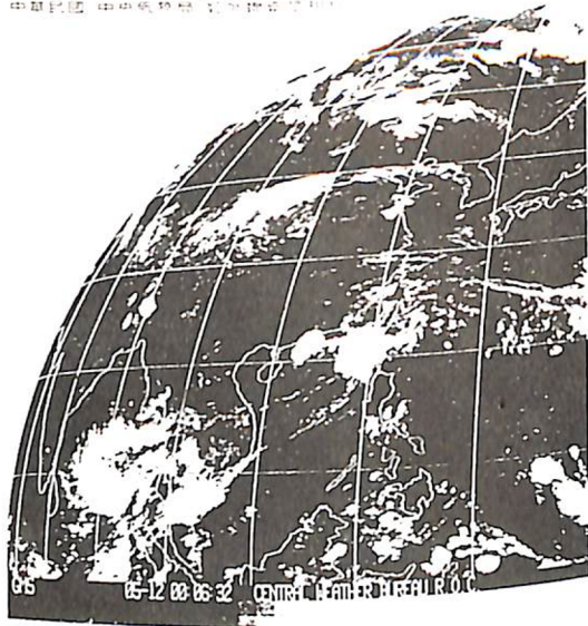
圖2-7 1986年5月12日00Z
