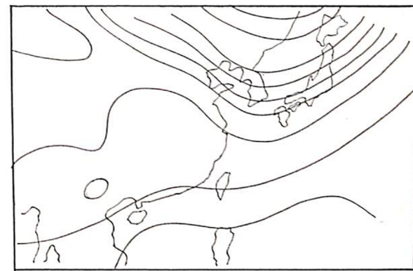
圖 7-3 5月11日 00 Z 700 mb 天氣圖
