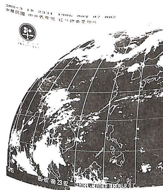
圖 2-2 1986年5月7日00Z
