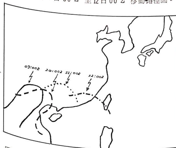
圖4 500 mb 5月9日至12日-5°C溫度脊移動路徑。
