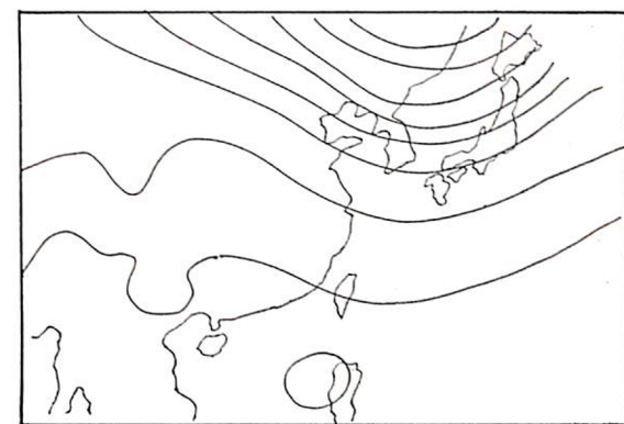
圖 8-3 5月11日 00 Z 500 mb 天氣圖
