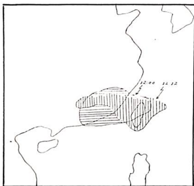
圖 5-4 5月12日 00 Z 及 12 Z
