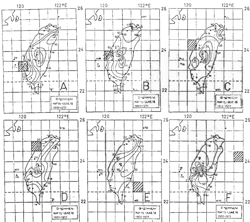
圖 7. 同圖 6, 但為小雨 (0.1 ~ 5.0 公厘 / 6 時) 之降水機率分布。
