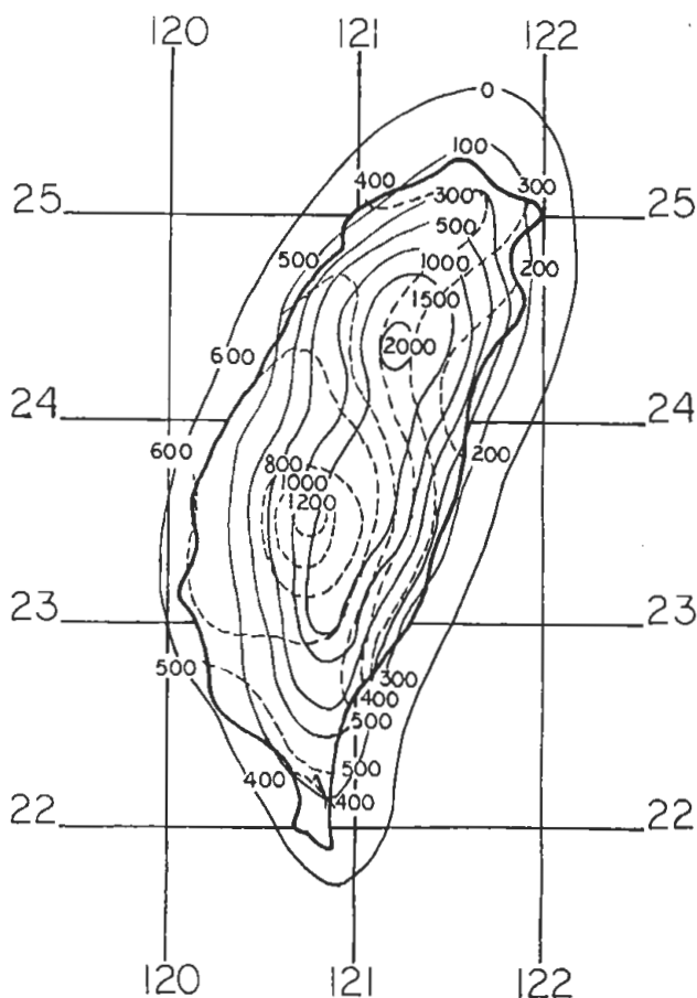
圖 10. 民國 61 年至 66 年（1972～1977）5 月 15 日至 6 月 18 日期間總降水量之年平均値分布。虛線為等雨量（公厘）實線為勻滑地形等高線（公尺）（採自陳，1978）。
