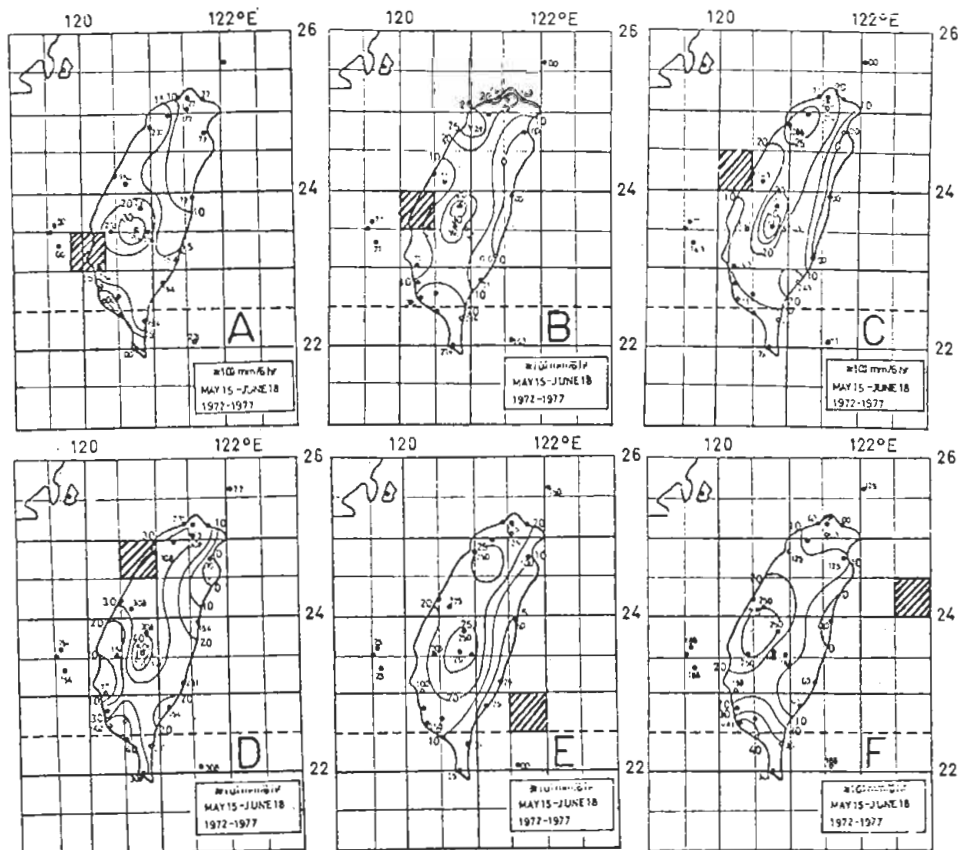
圖 9. 同圖 6，但為大雨（≥ 10.1 公厘 / 6 時）之降水機率分布。
