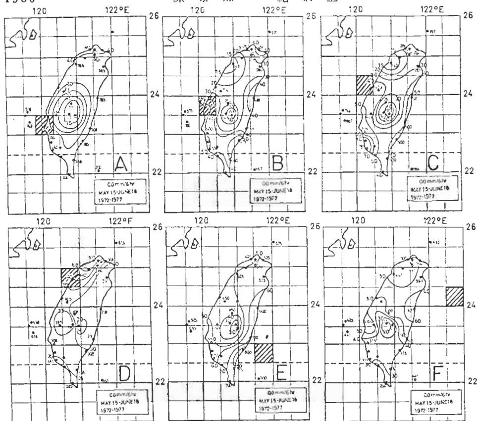
圖 6. 民國 61 年至 66 年 (1972 ~ 1977) 5 月 15 日至 6 月 18 日 間中幅度低壓出現於斜線方塊時各地無雨 (0.0 公厘 / 6 時) 之降水機率分布。
