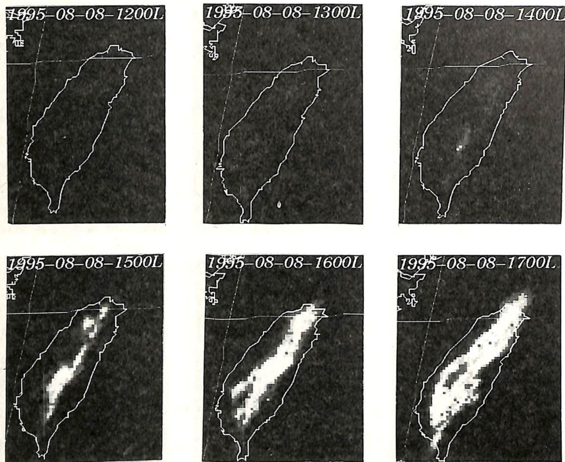
圖 6：1995年8月8日之IRIS雲圖。
