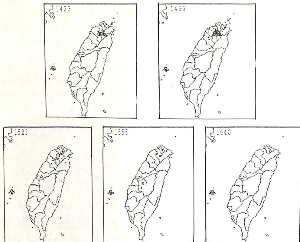
圖 4：1994年8月23日1423至1640時各前30分鐘內之落雷資料。
