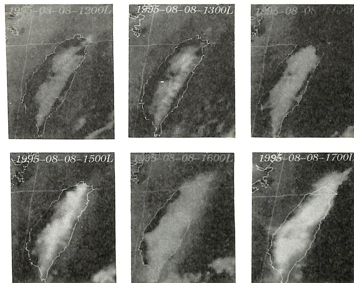
圖 5：1995年8月8日之紅外線雲圖。
