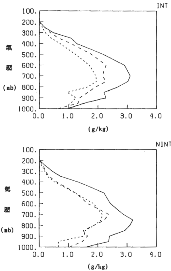
圖 7. 0-2°混合比偏差值 ( q' )。INT 表加強型，NINT 表非加強型，實線為STAGE 2，點線為STAGE 0，虛線為STAGE 1，實線為STAGE 2。(單位 g/kg)
