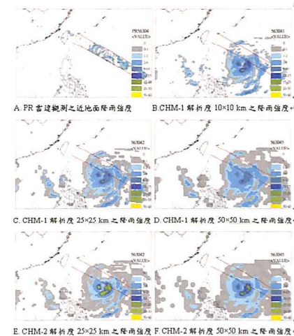
圖 3.1 2007 年 10 月 3 日 0940-0946 UTC 降降雨強度分布圖。
