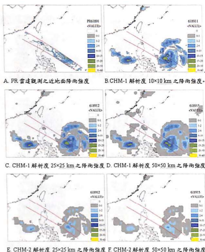
圖 3.3 2008 年 9 月 25 日 2044-2053 UTC 降雨強度分布圖
