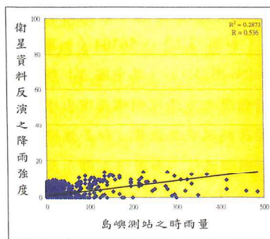
圖 3.4 2007 年柯羅莎颱風通過島嶼測站時衛星資料反演之降雨強度與島嶼地面雨量計之累積雨量對照圖。
