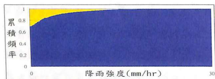
圖 2.4 2009/08/05 0530 UTC 莫拉克颱風之降雨強度累積直方圖。
