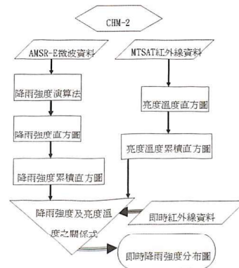
圖2.3 CHM-2降雨量估計流程圖。
