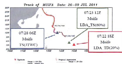
圖 3 個案 112011 梅花颱風的 JTWC 發佈 TS 及 LDA 60% 之位置圖。
