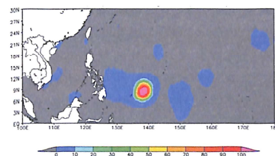
圖1 颱風發展機率示意圖。不同的顏色代表不同的發展機率，單位為%。
