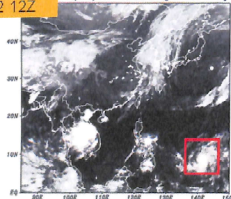
圖6 案012015紅霞颱風於2015年5月2日1200 UTC的IRI雲圖、方框代表當時紅霞颱風的位置。
