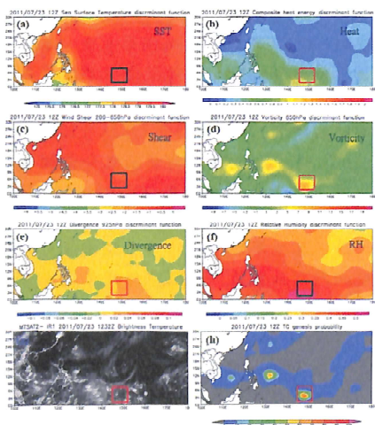
圖 4 個案 112011 梅花颱風於 2011 年 7 月 23 日 1200 UTC 的(a)-(f)各參數判別函數分佈圖、(g)IR1 雲圖、(h)潛勢機率分佈圖，方框代表當時梅花颱風的位置。
