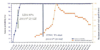
圖2 個案 112011 梅花颱風的最大維持風速(橘色)與潛勢發展機率(藍色)時序圖。
